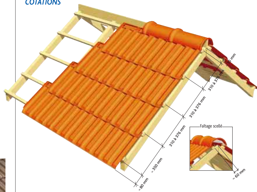
Pose avec rives individuelles
