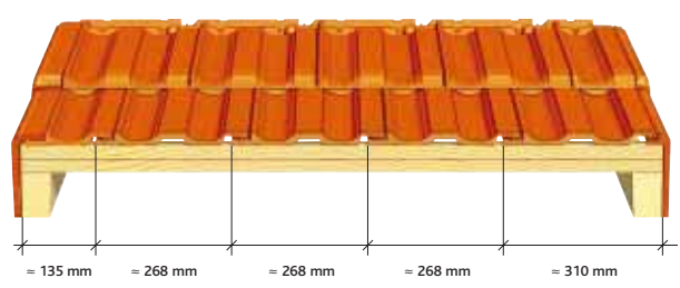
Pose avec rives individuelles
